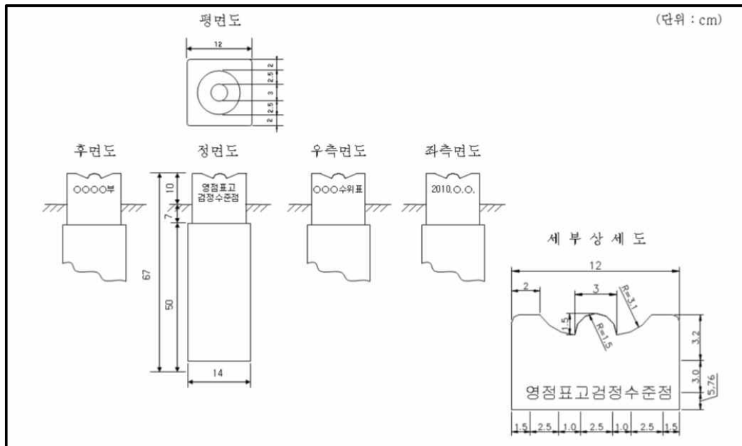
< 영점표고검정수준점 표준규격 >
